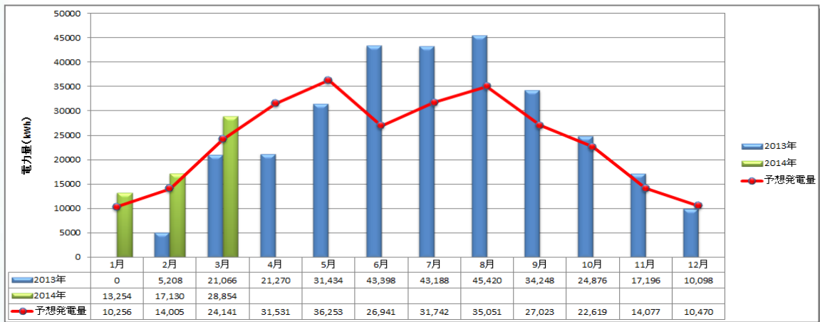
[発電実績(平成 25 年 2 月～平成 26 年 3 月末)]
